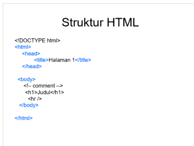
Gambar 3 . 2 Struktur dari HTML
