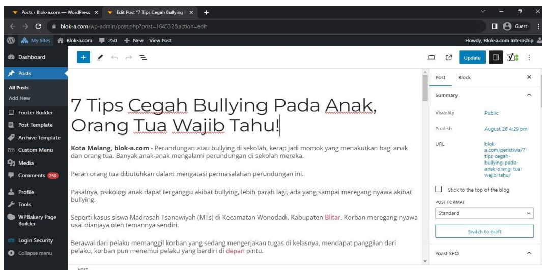
Gambar 3.6 Tampilan Edit-Post
