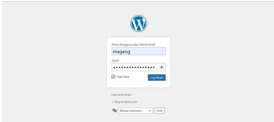
Gambar 3.3 Tampilan Login
