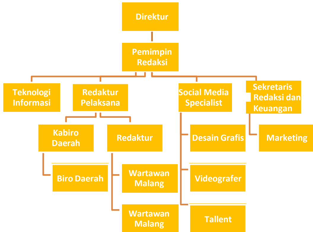
Gambar 2.1 Struktur Blok-a.com
