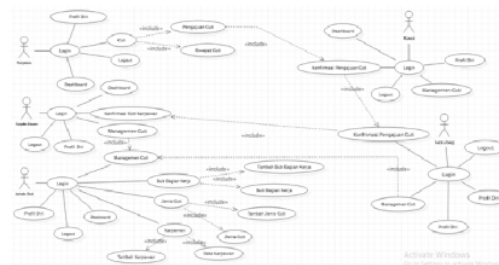
Gambar 2 Use Case Diagram Sistem Informasi Cuti
