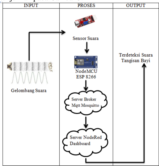
Gambar 3. Blok Diagram yang diusulkan
